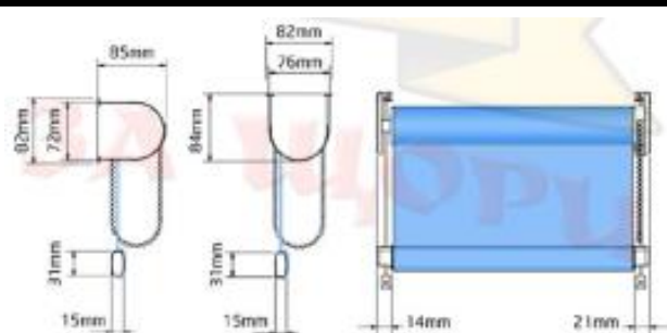
Dimensiuni console sistem 40+
