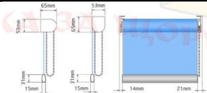
Dimensiuni console sistem Comfort
